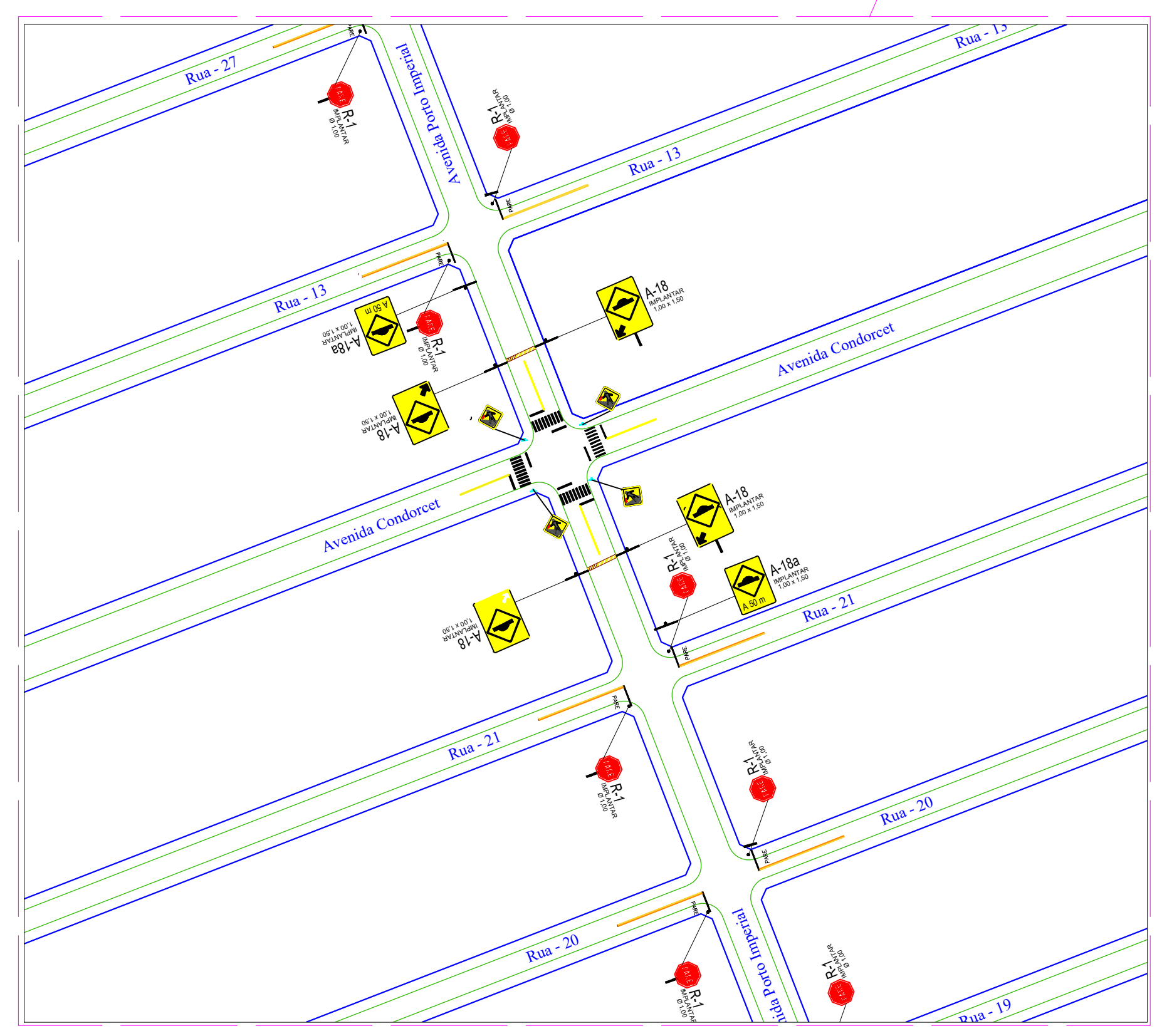
1 PLANTA BAIXA DE IMPLANTAÇÃO DE SINALIZADORES VIÁRIOS ESCALAS sem escala
